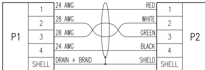
WIRING TABLE
